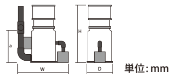
外形寸法図 プロテインスキマー内部式モデル
